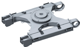
대형 하부 프레임 Lower Frame_large
