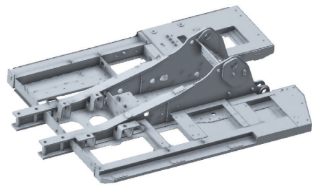
상부 Main Frame
