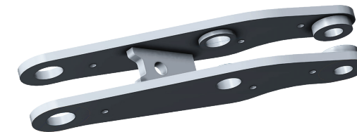
벨크랭크 Bellcrank
