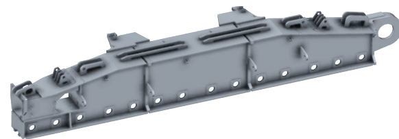
크롤러 프레임 Crawler Frame
